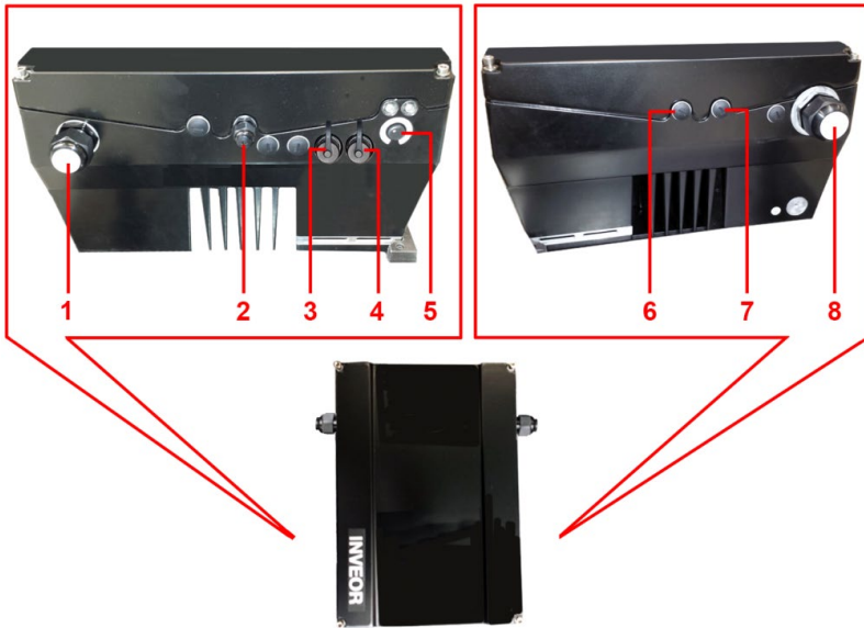
Abb.: 7 Anschlüsse BG. D „PROFIBUS“
