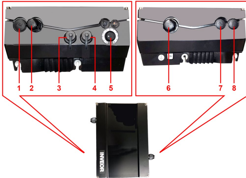
Abb.: 5 Anschlüsse BG. A „PROFIBUS“
