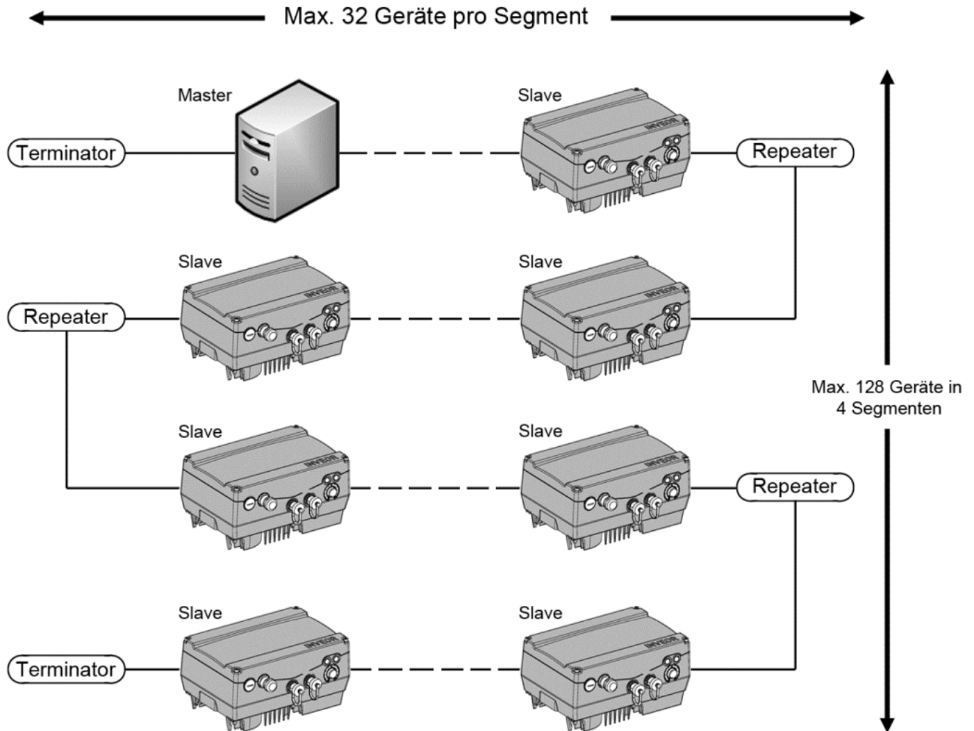
Abb.: 4 Verkabelung und Busanschluss
