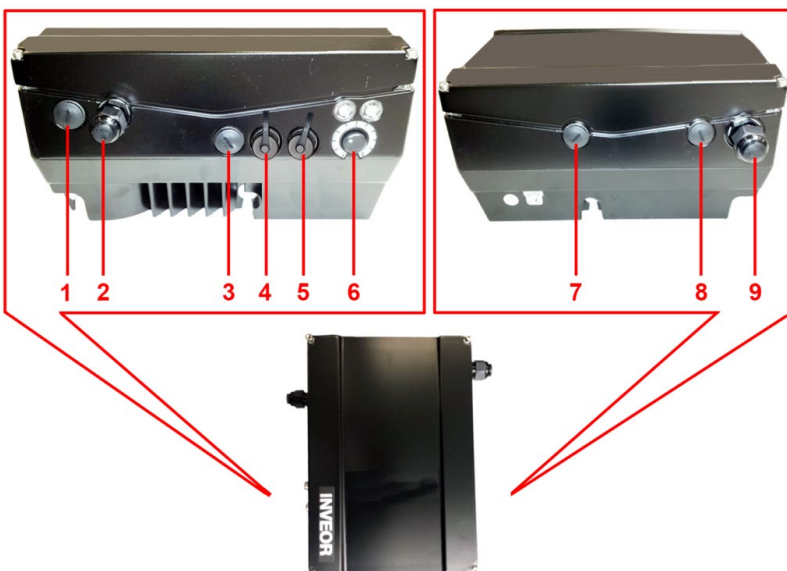
Abb.: 6 Anschlüsse BG. B - C „PROFIBUS“
