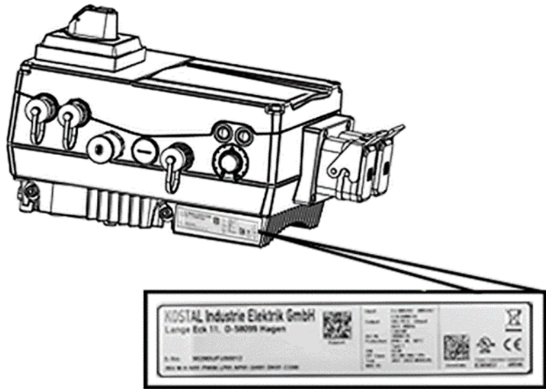
Abb. 4: Kennzeichnungen am Antriebsregler
