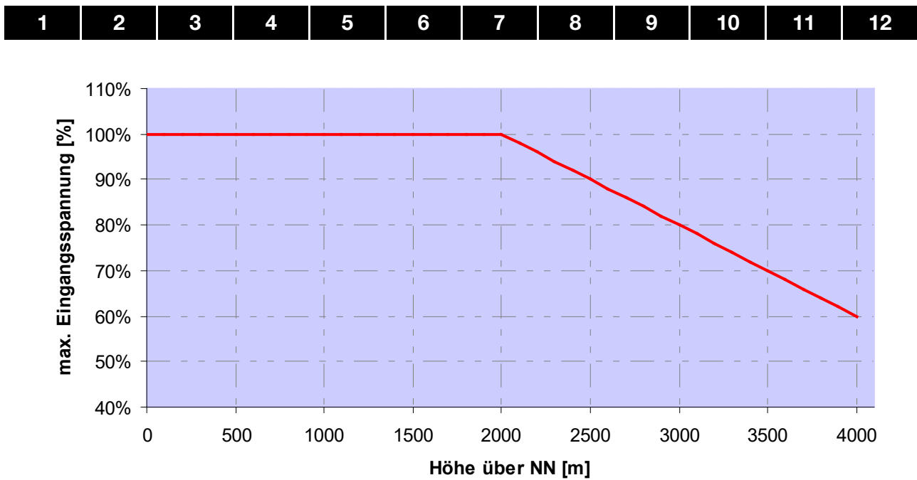
Abb. 56: Derating der maximalen Eingangsspannung aufgrund der Aufstellhöhe
