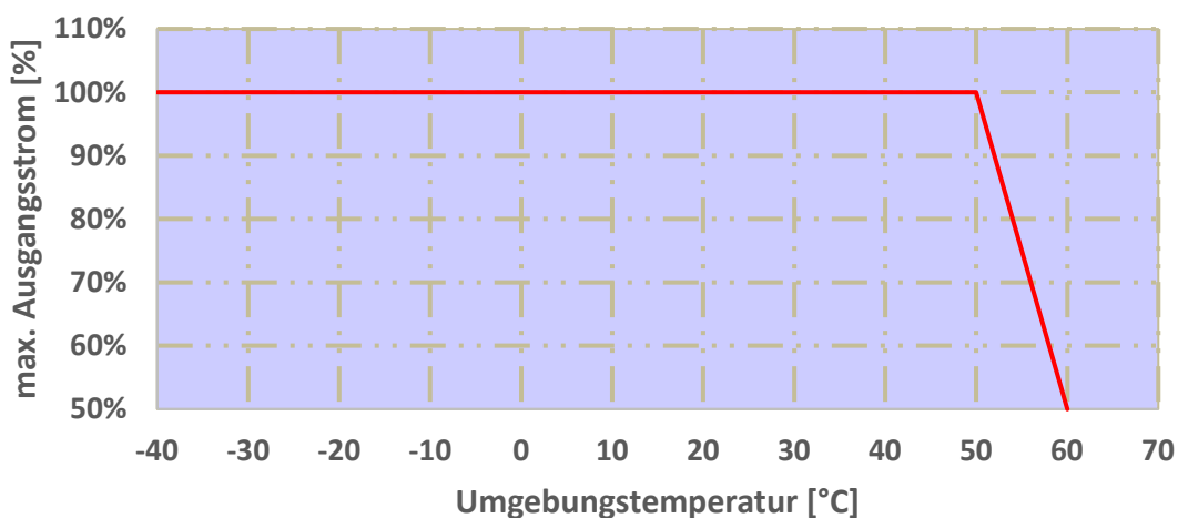
Abb. 53: Derating für motormontierte Antriebsregler
