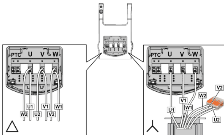
Abb. 12: Stern- oder Dreieck-Schaltung BG A
