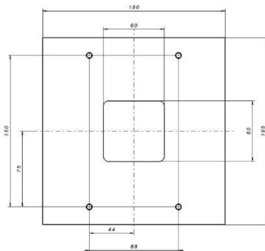
Abb. 61: Bohrbild Standard-Adapterplatte BG D
