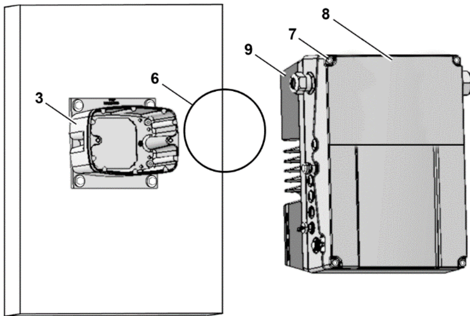
Abb. 40: Einsetzen der O-Ring-Dichtung BG. D
