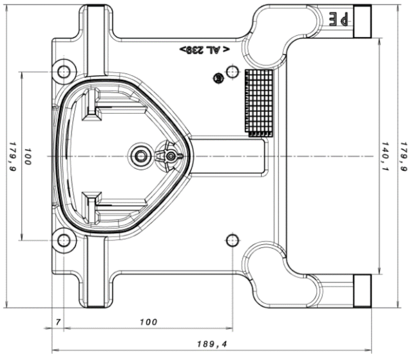
Abb. 64: Bohrbild Standard-Wand-Adapterplatte BG C
