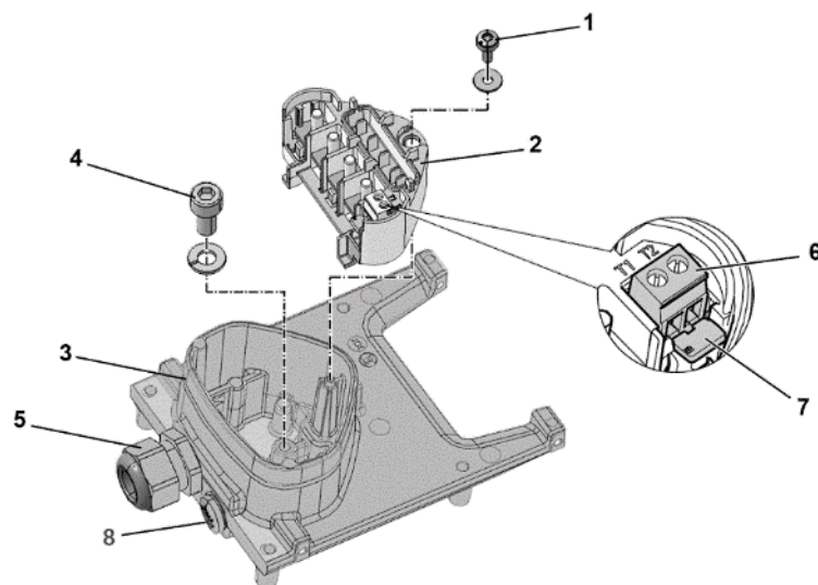
Abb. 37: Verdrahtung Wandadapterplatte BG. B-C
