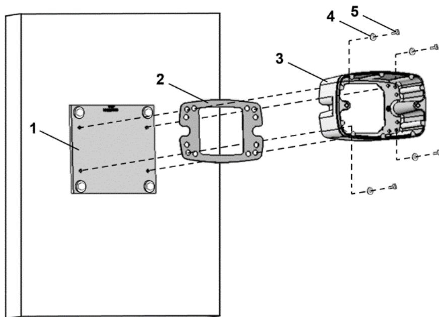
Abb. 39: Befestigung des Becher BG. D an der Adapterplatte
