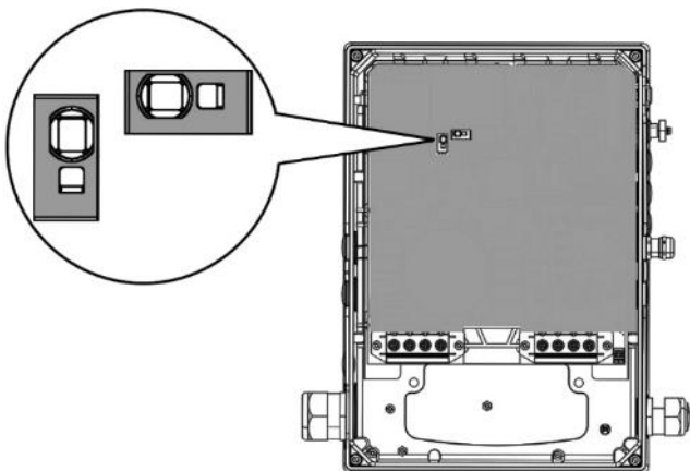
Abb. 18: Baugröße D
