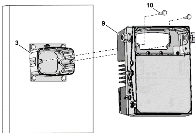
Abb. 41: Befestigung Antriebsregler auf Becher BG. D
