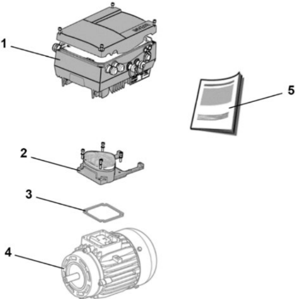
Abb. 6: Lieferumfang
