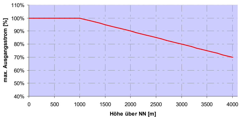
Abb. 55: Derating des maximalen Ausgangsstrom aufgrund der Aufstellhöhe
