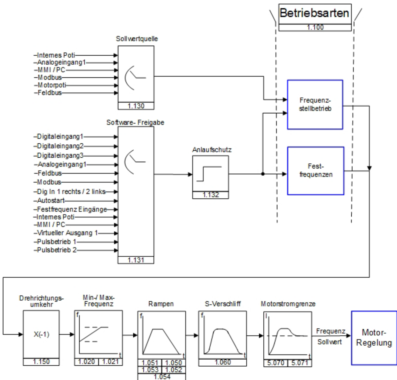
Abb. 51: Allgemeine Struktur Sollwertgenerierung
