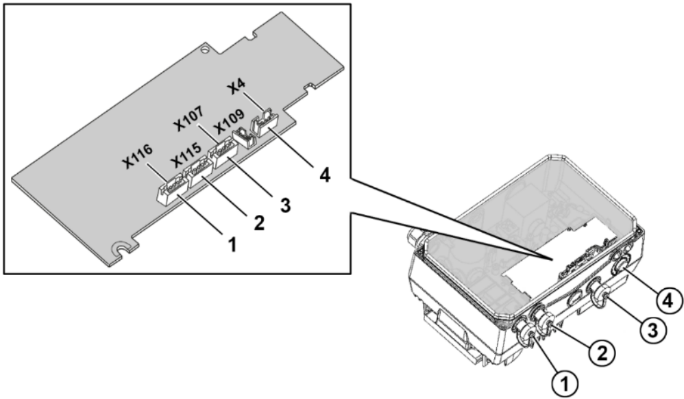
Abb. 26: IO Modul / Belegung der Stecker (Option)
