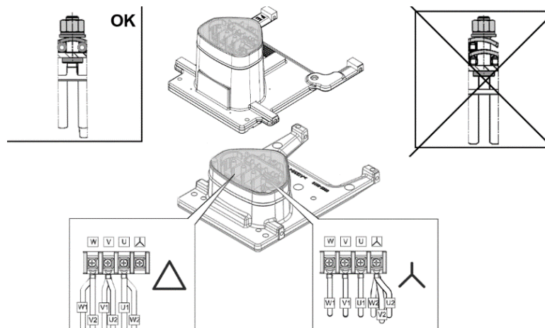
Abb. 13: Stern- oder Dreieck-Schaltung BG B-C
