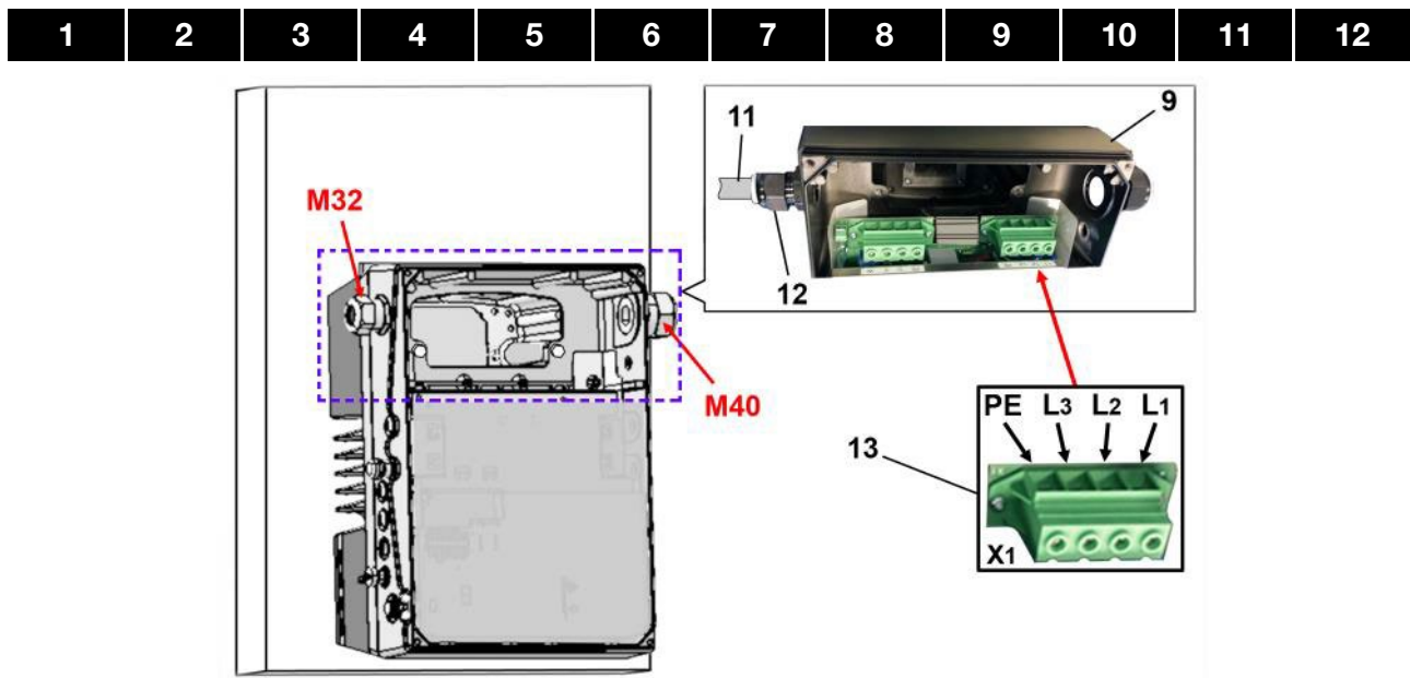
Abb. 42: Netzanschluss BG. D
