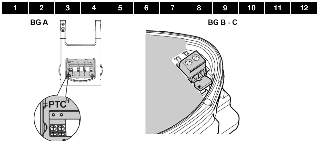
Abb. 15: Einlegebrücke
