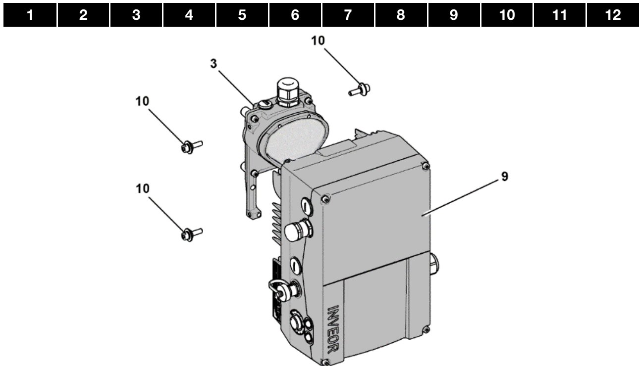
Abb. 38: Antriebsregler aufsetzen
