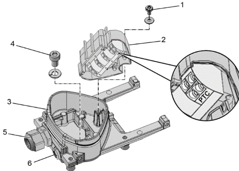
Abb. 35: Verdrahtung Wandadapterplatte BG. A
