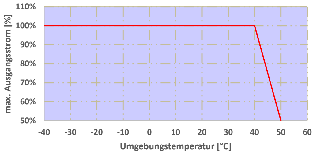
Abb. 54: Derating für wandmontierte Antriebsregler
