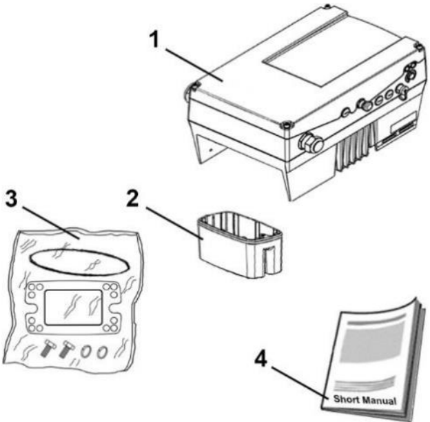
Abb. 7: Lieferumfang BG. D
