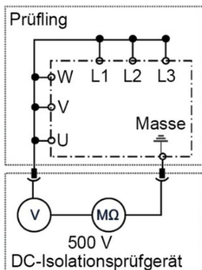
Abb. 5: Isolationsprüfung am Leistungsteil
