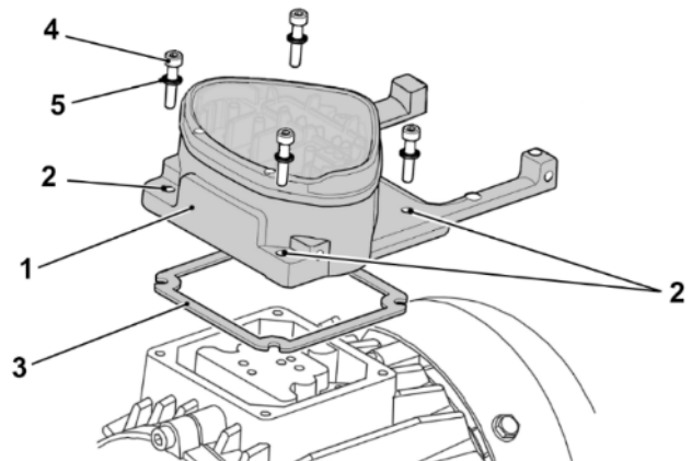
Abb. 14: Reihenfolge Zusammenbau: Anschlusskasten – Adapterplatte (BG A - C)
