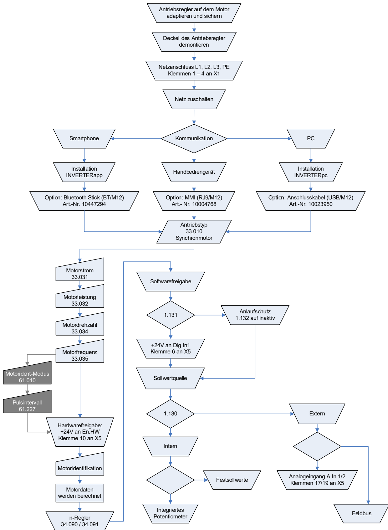
Abb. 68: Blockdiagramm Schnellinbetriebnahme PMSM und SynRN
