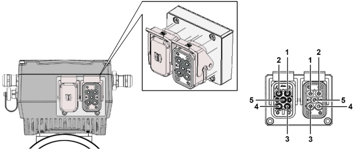
Abb. 19: Harting -Stecker
