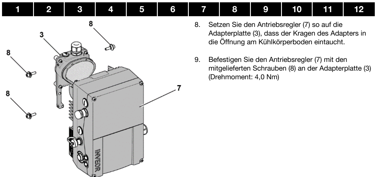
Abb. 36: Antriebsregler aufsetzen
