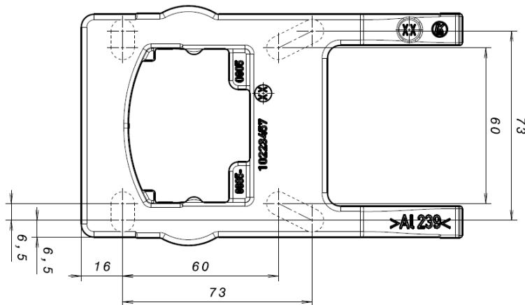
Abb. 58: Bohrbild Standard-Adapterplatte BG A
