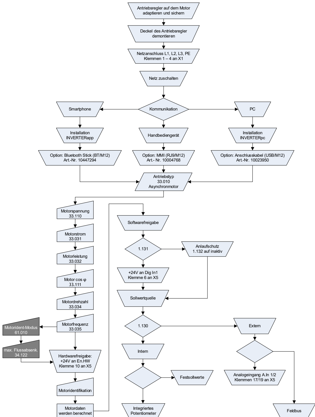
Abb. 67: Blockdiagramm Schnellinbetriebnahme ASM
