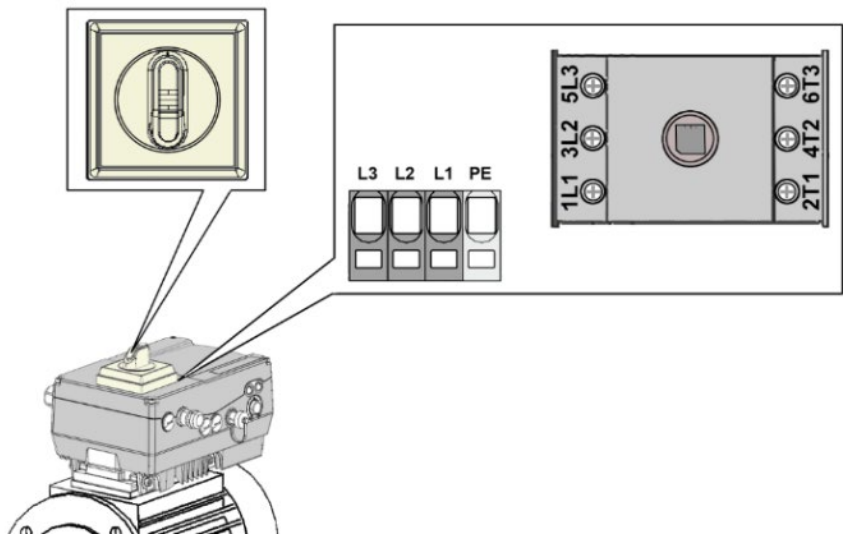
Abb. 21: Hauptschalter
