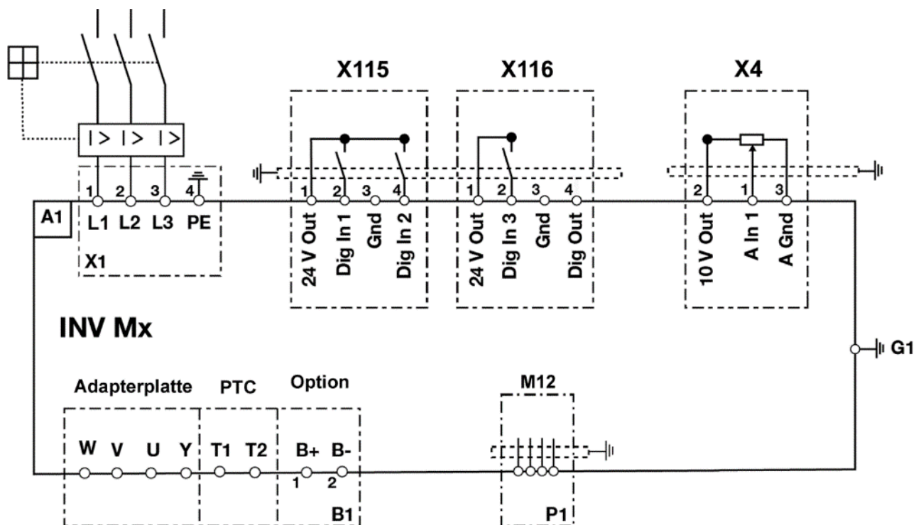
Abb. 22: Anschlussplan (Option IO Modul)
