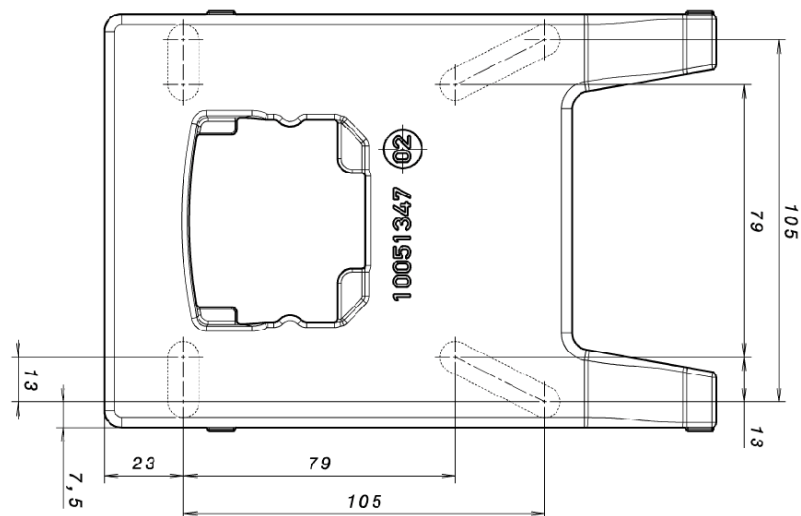
Abb. 59: Bohrbild Standard-Adapterplatte BG B
