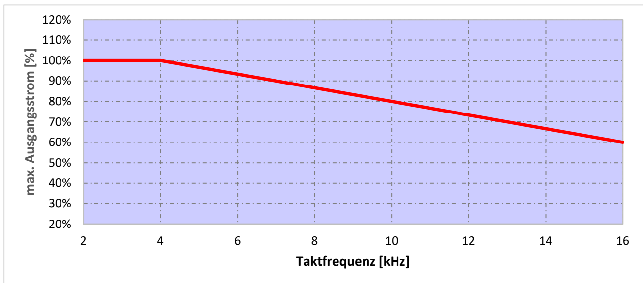
Abb. 57: Derating des maximalen Ausgangsstroms aufgrund der Taktfrequenz
