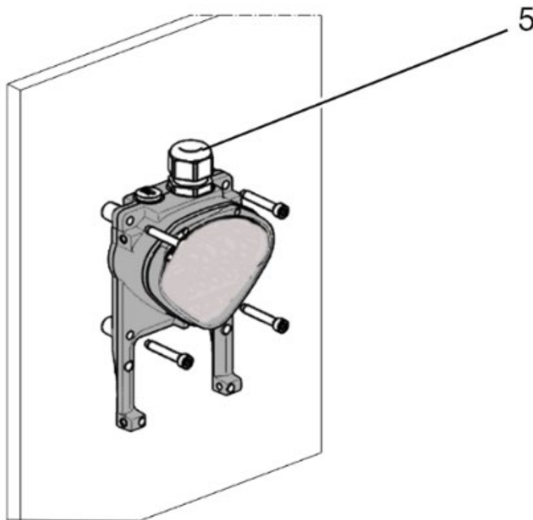
Abb. 34: Befestigung der Adapterplatte an der Wand
