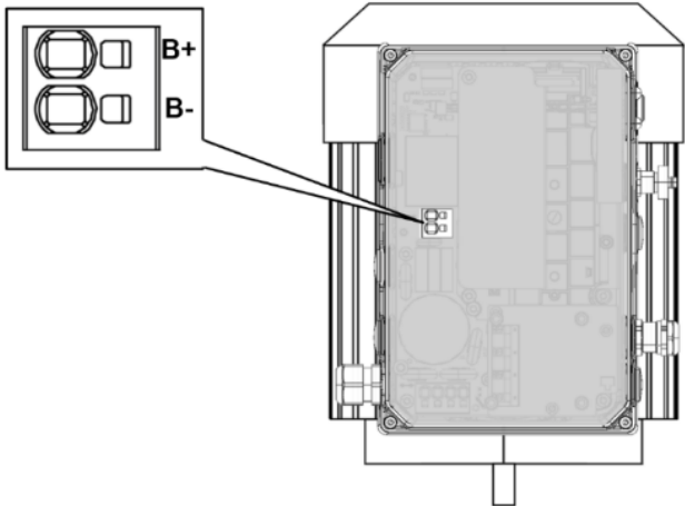
Abb. 17: Baugröße A - C
