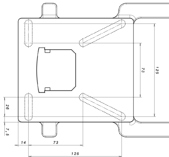
Abb. 60: Bohrbild Standard-Adapterplatte BG C
