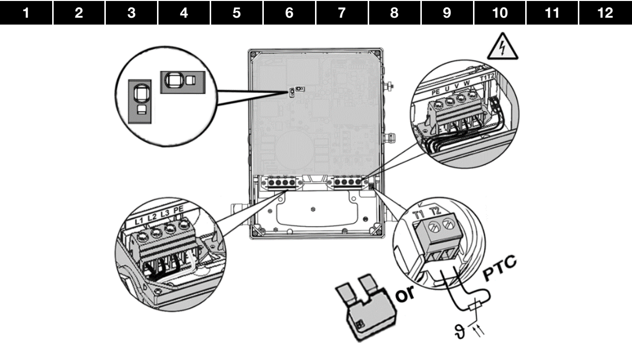
Abb. 16: Baugröße D
