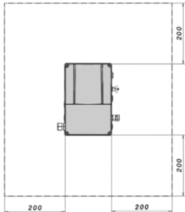
Abb. 32: Mindestabstände
