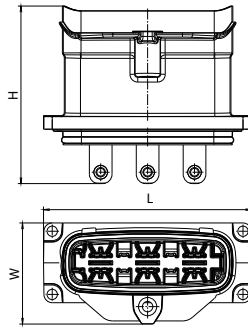
Tab Header 180 °
