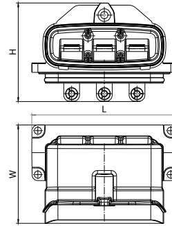
Tab Header 90 °
